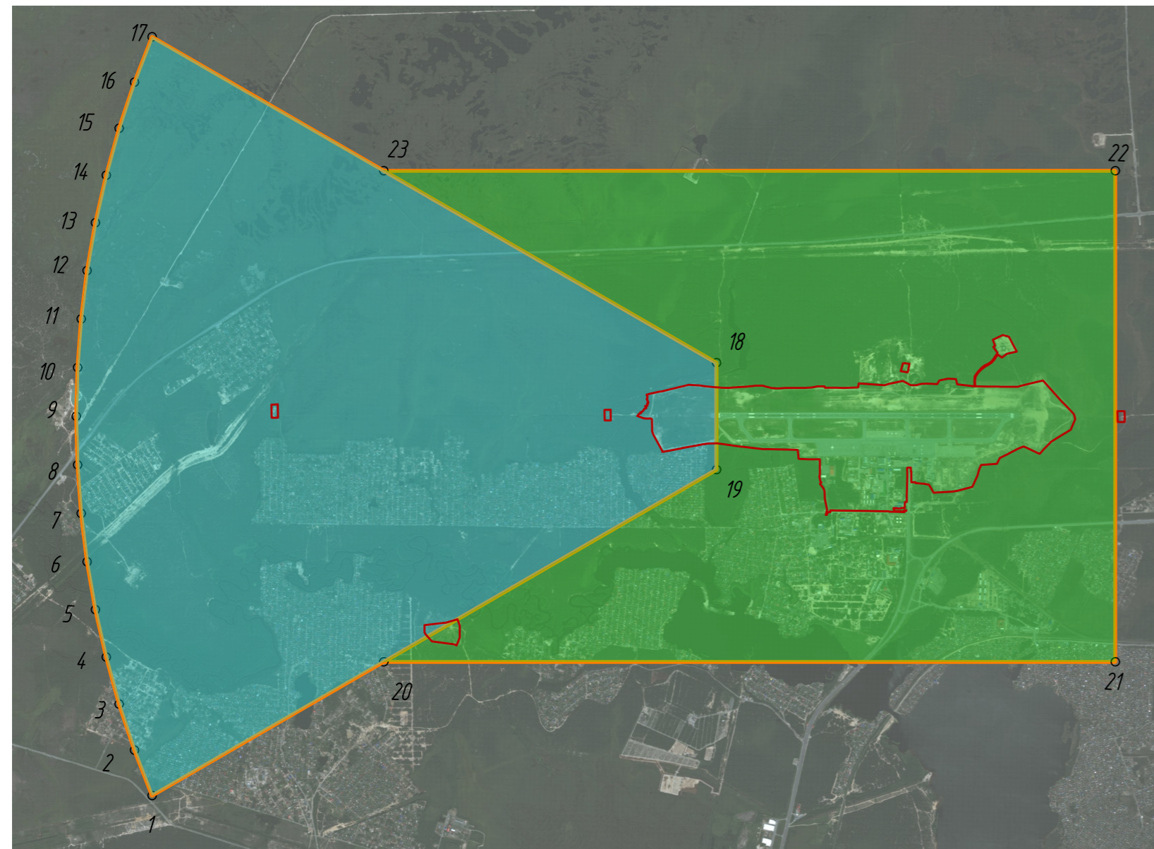
Защитные зоны КРМ-73
